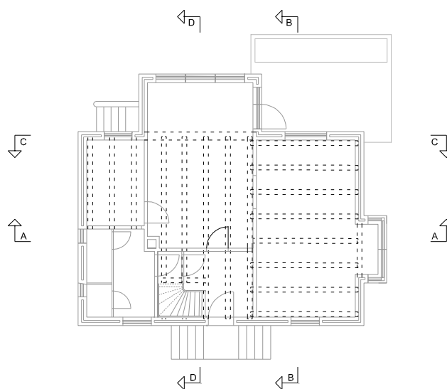
Stueetage
